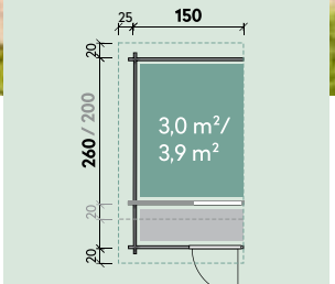
Anbauschuppen 1520/1526
